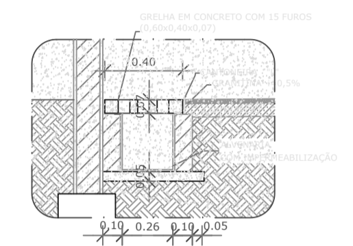
1 DETALHE 1: CALHA DE PISO ESCALA 1/25
