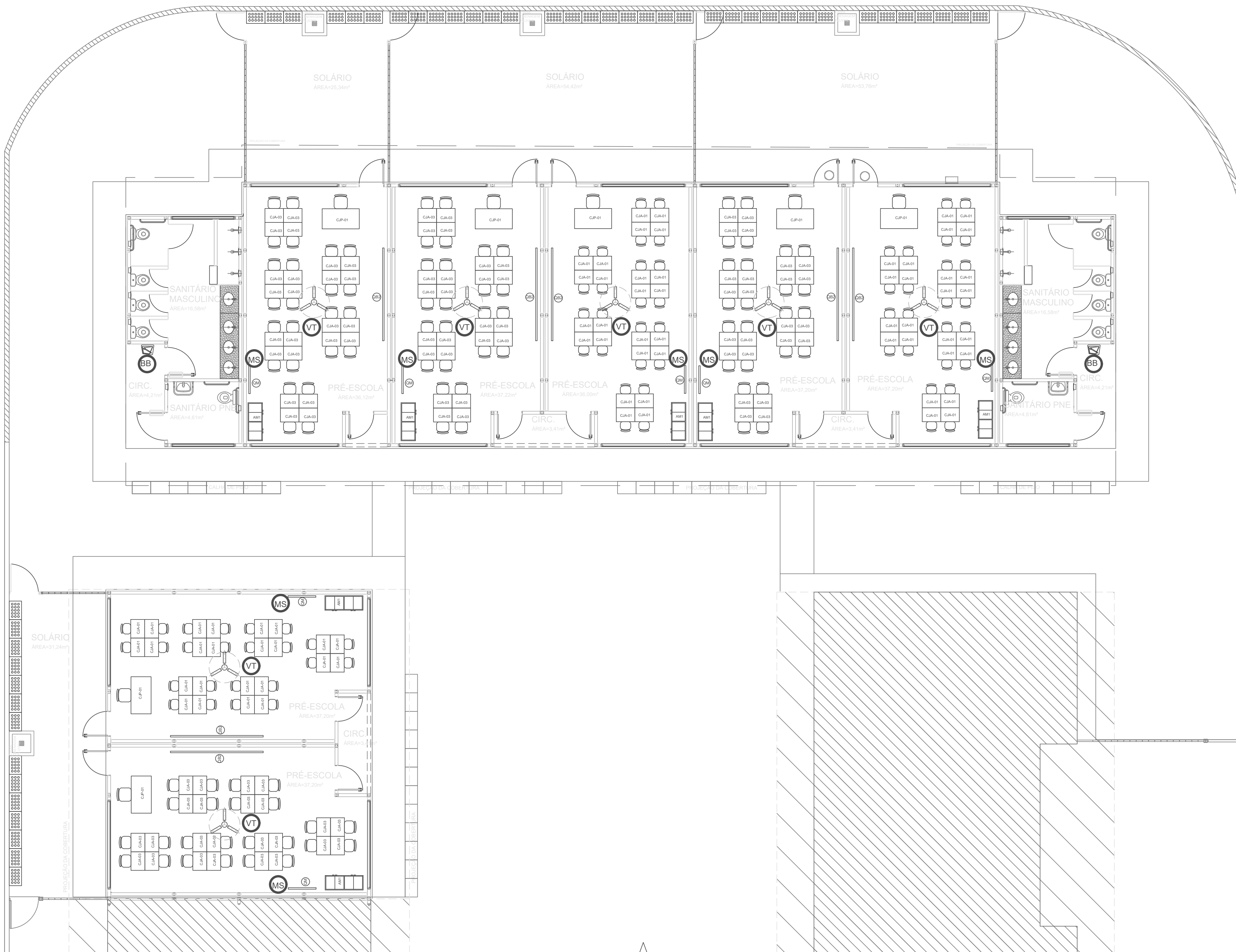
1 PLANTA BAIXA ESCALA 1/75
