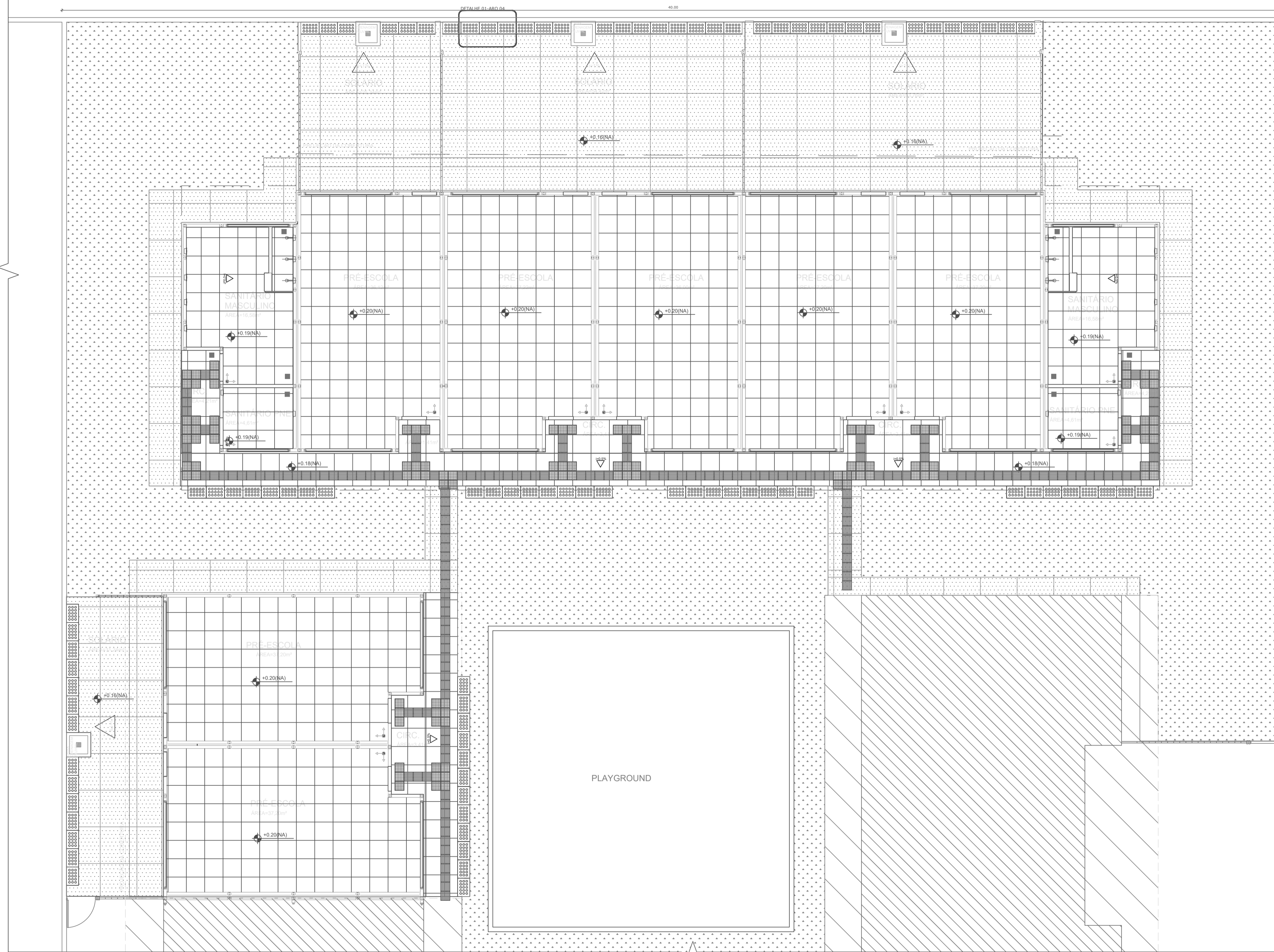
1 PLANTA DE PAGINAÇÃO DE PISO ESCALA 1/50
