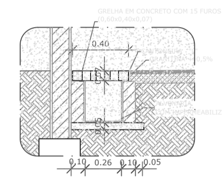
1 DETALHE 1: CALHA DE PISO ESCALA 1/25
