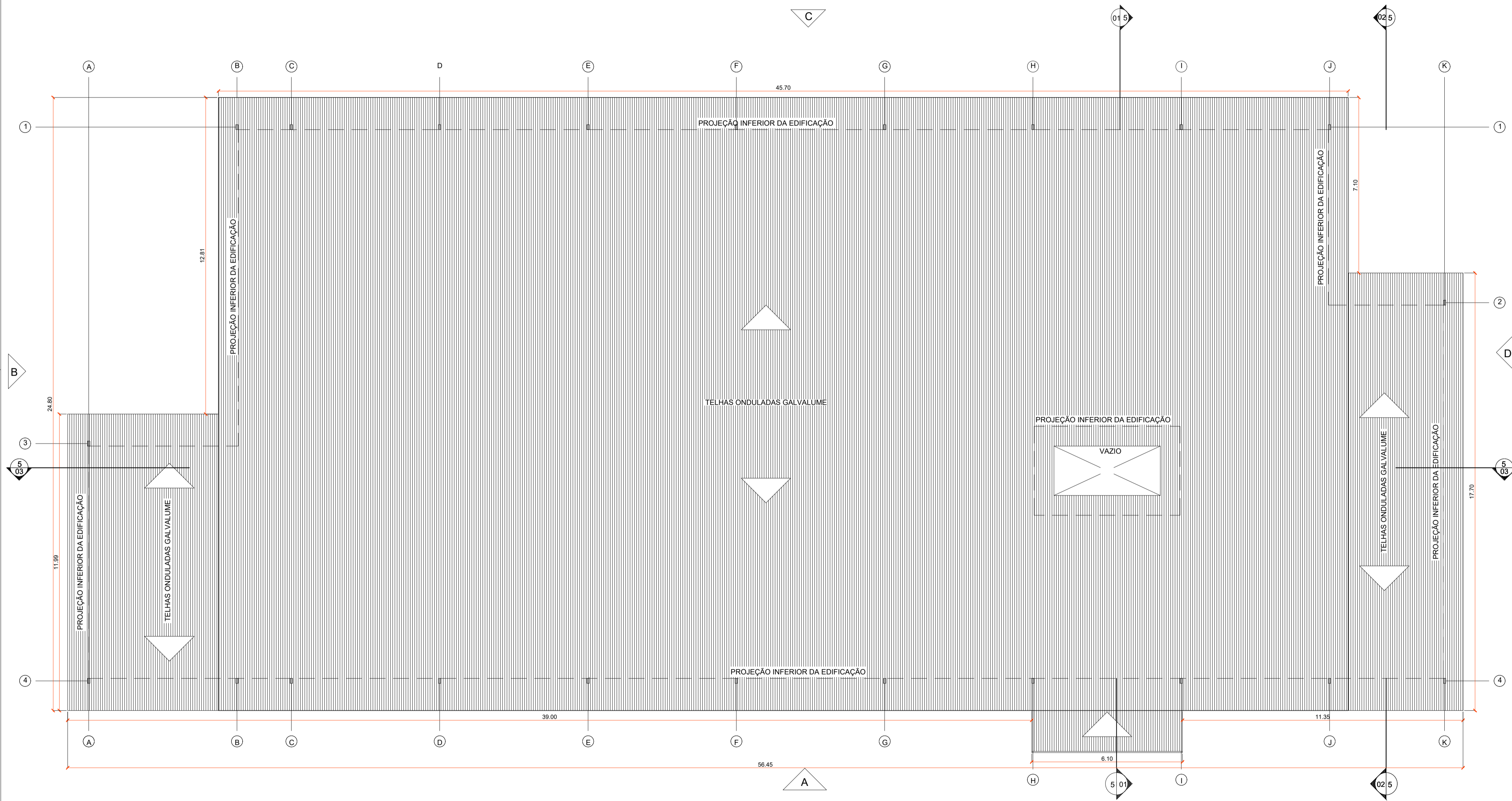
1 PLANTA DE TELHADO ESC:1/100
